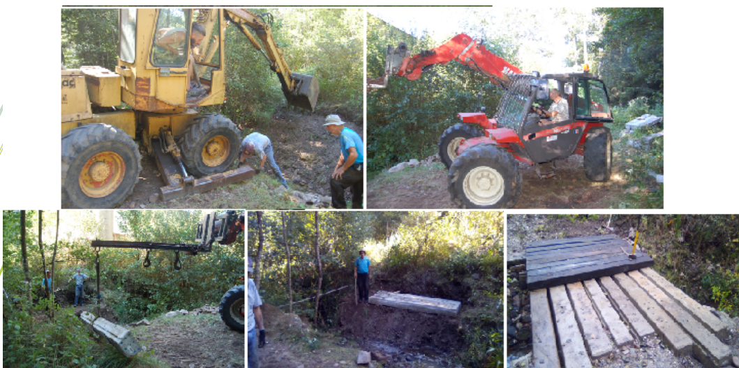
Passerelle du "Clou-Atre"
